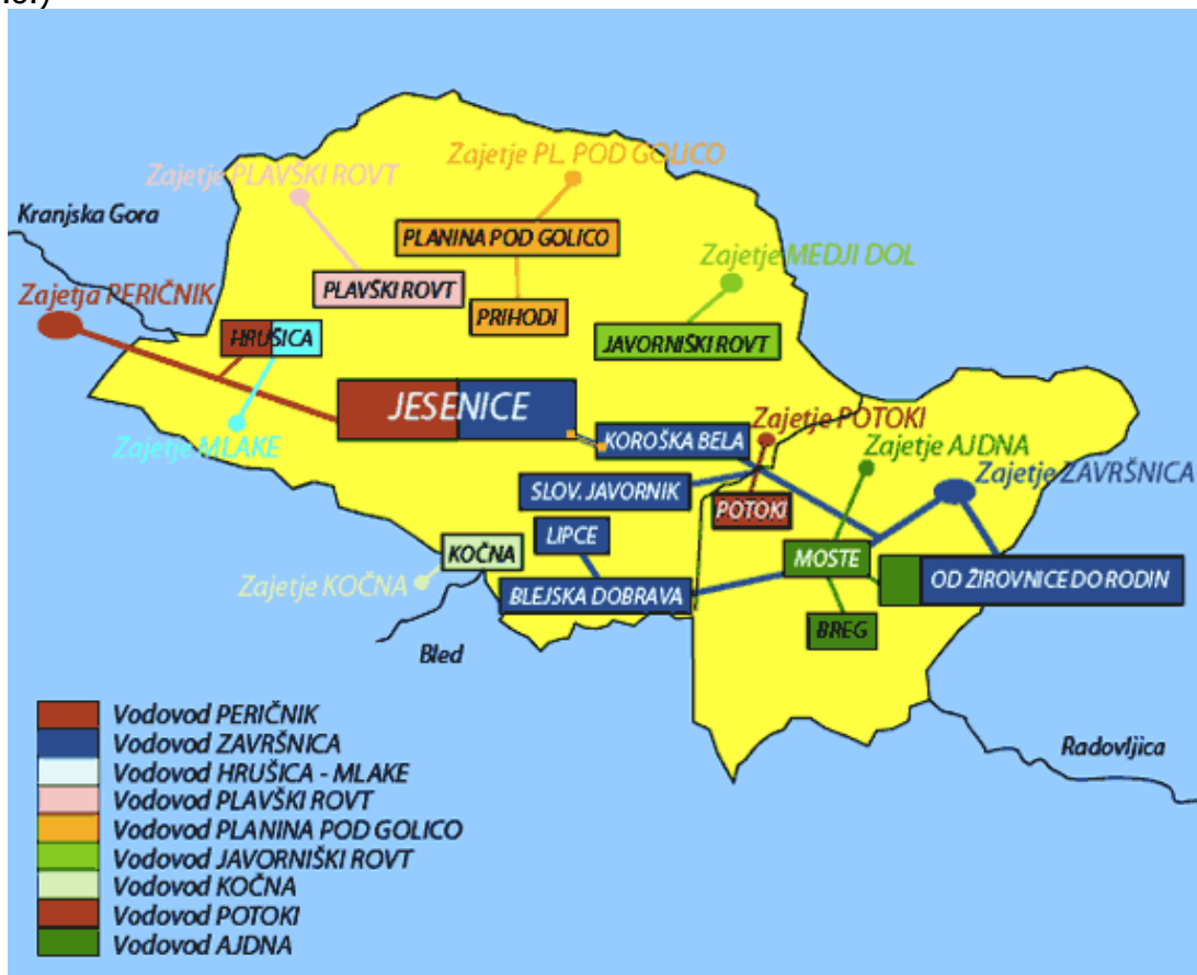
Slika 1: Shema cevovodov v občini Žirovnica in občini Jesenice (Vir: JEKO-IN, d.o.o.)
